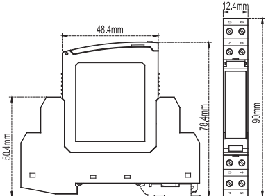
外形尺寸
