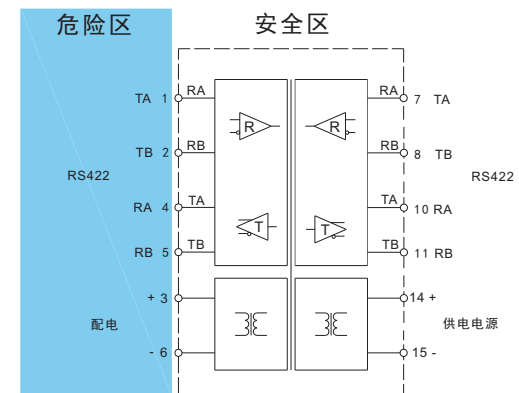
RS422输入RS422输出
