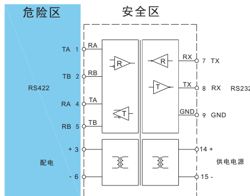
RS422输入RS232输出
