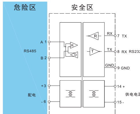
RS485输入RS232输出
