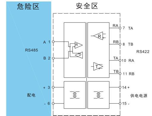
RS485输入RS422输出
