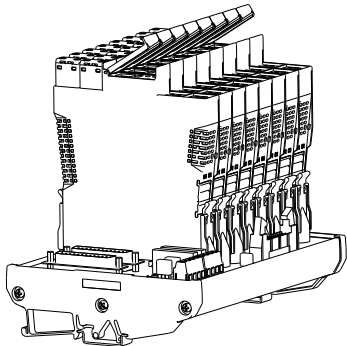
安装示意图
