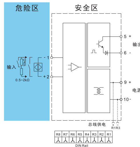
单入单出接线图
