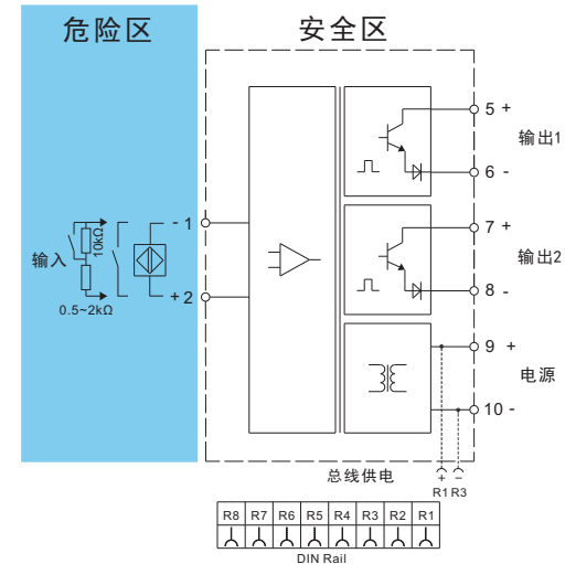
单入双出接线图
