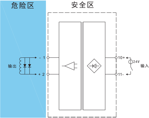
单入单出接线图
