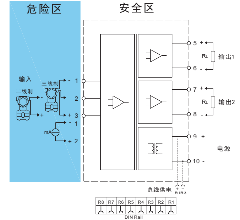
单入双出接线图
