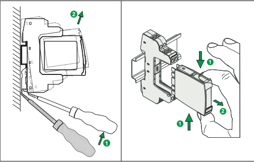
拆卸步骤图
