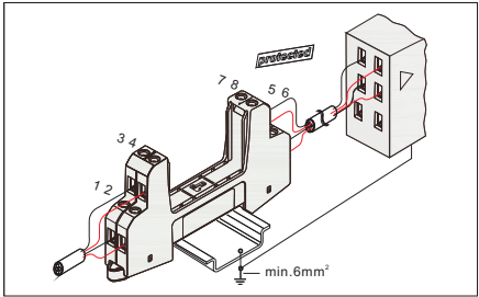
连接示意图
