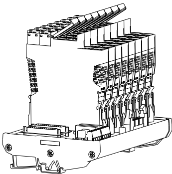
安装示意图
