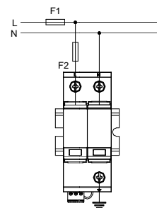
单相 TT 系统
