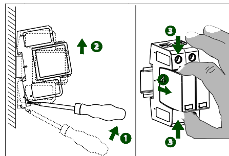
拆卸步骤图
