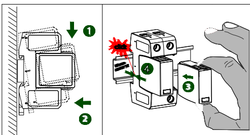
安装步骤图
